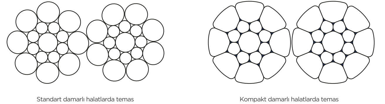
Şekil 11: Geleneksel ve kompakt halatlarda temas
