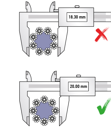
Şekil 5: Doğru ve yanlış çap ölçümü
